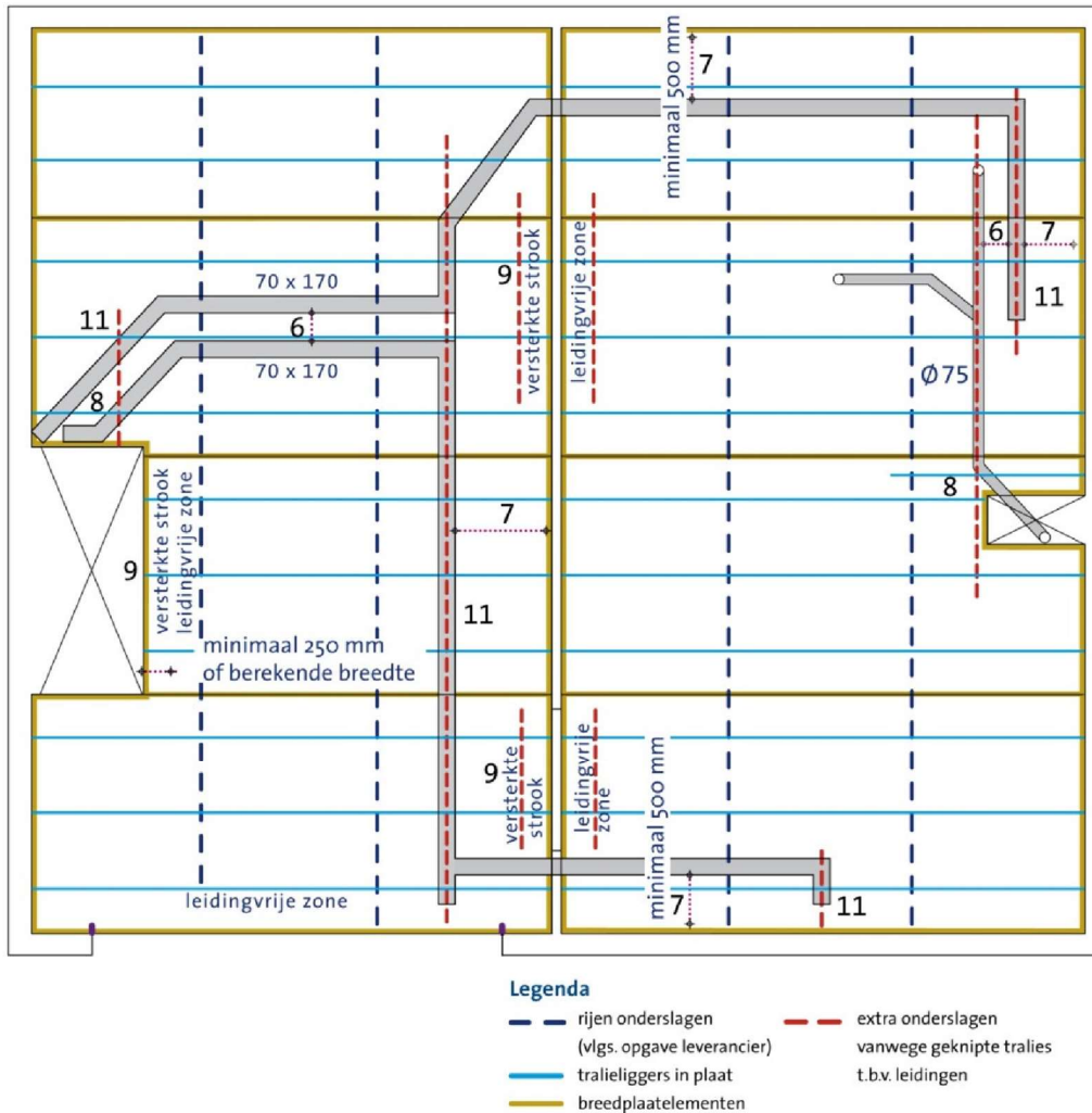
Figuur 2: Een voorbeeld plattegrond (vervolg legenda hierna)
